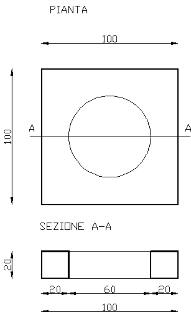
Figura 1: Geometria del manufatto
